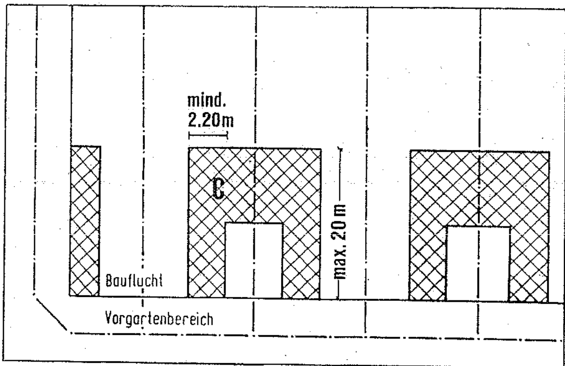
Abb. ÜBERGANGSBEREICH:
