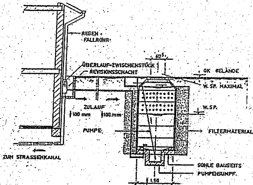
Abb. KOMBINIERTE REGENRÜCKHALTE- UND SICKERSCHACHTANLAGE:
